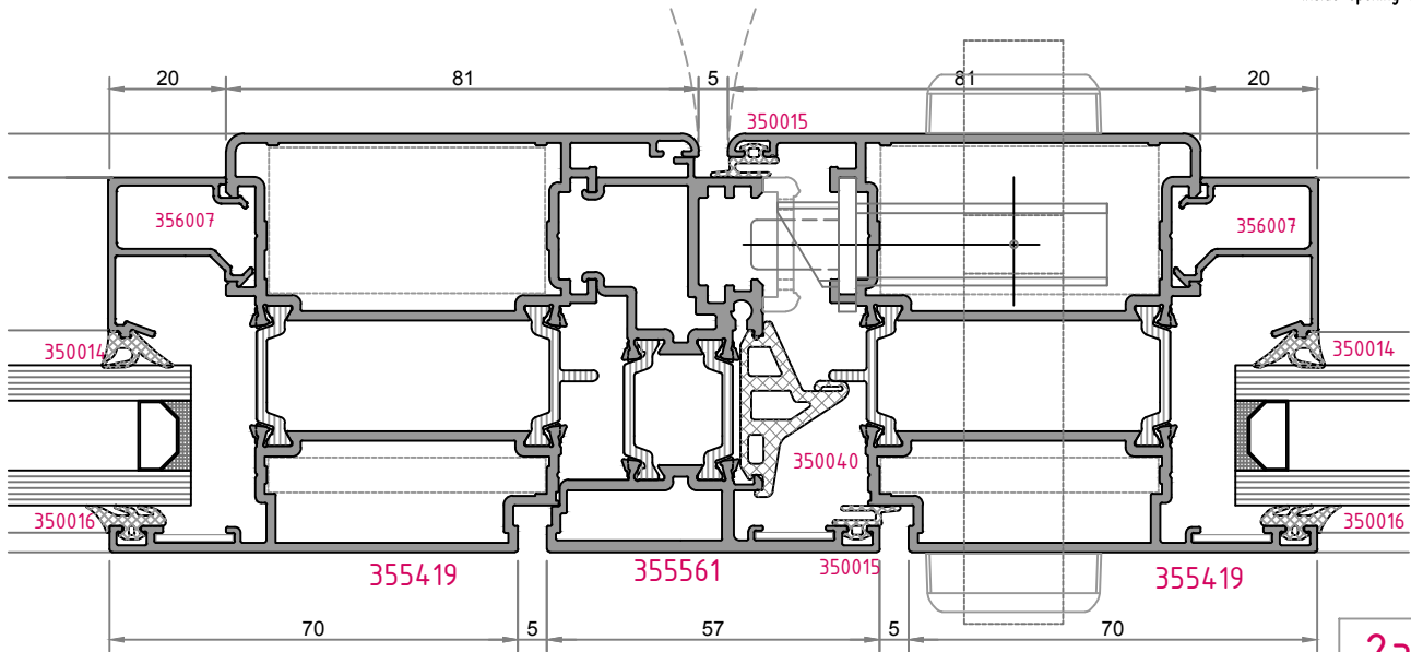
içe açılım kapı inside opening door
