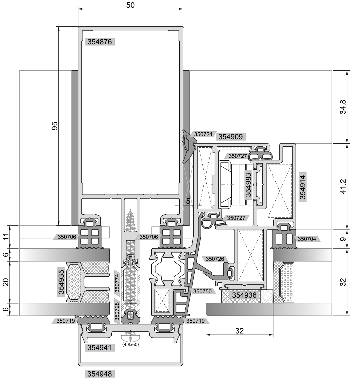
DÜŞEY DETAYI VERTICAL DETAIL
