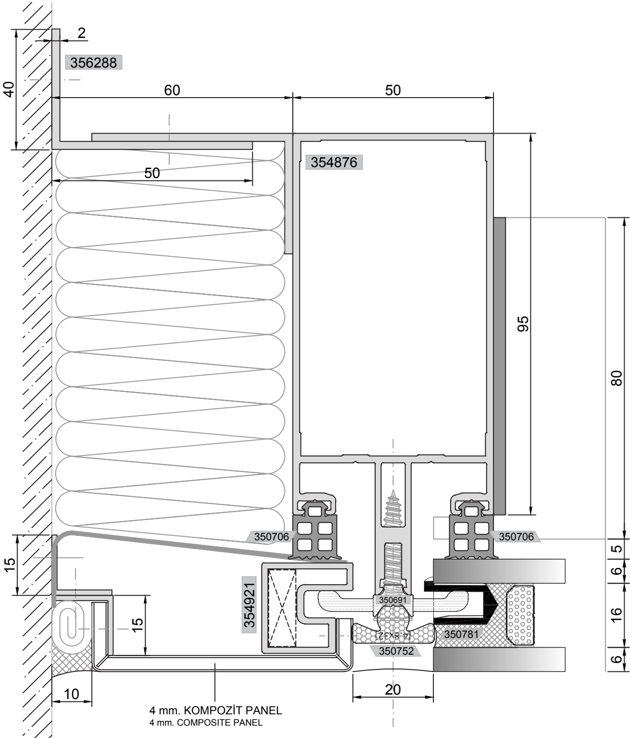
DÜŞEY DETAYI VERTICAL DETAIL
