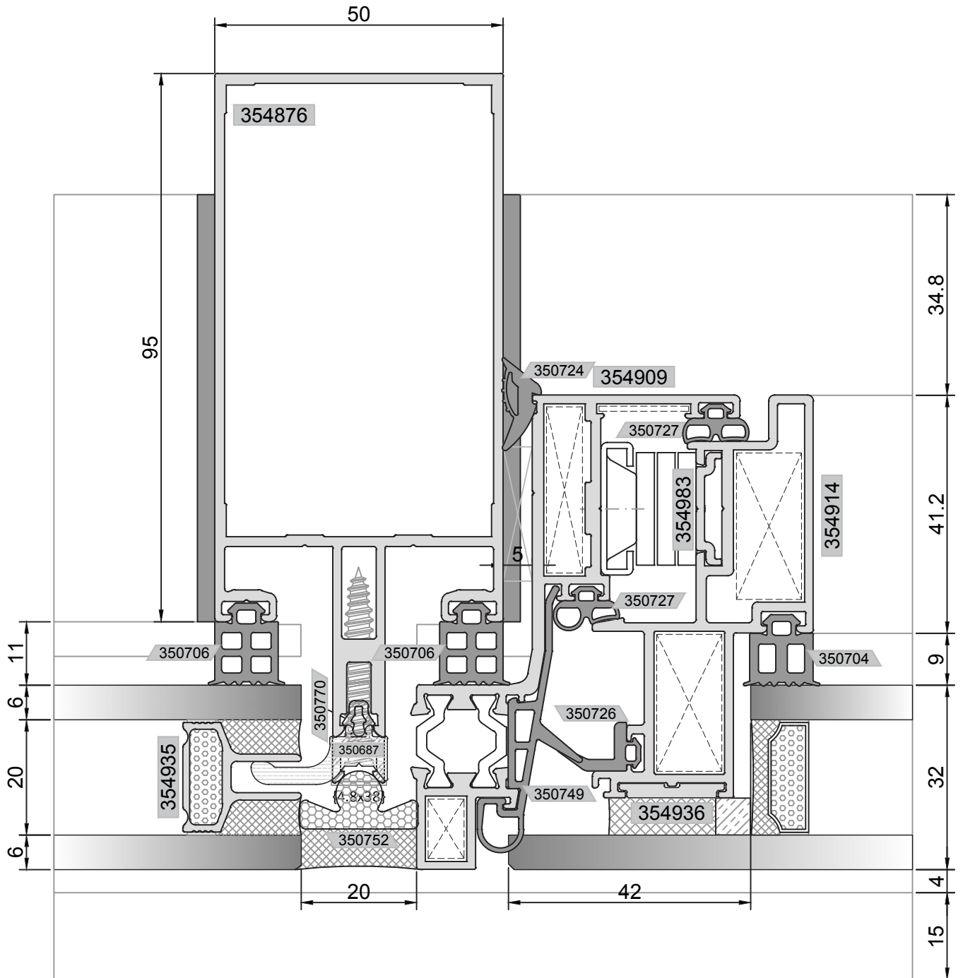
DÜŞEY DETAYI VERTICAL DETAIL
