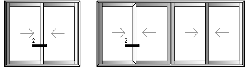
2 raylı sistem detayları Double rail system details
