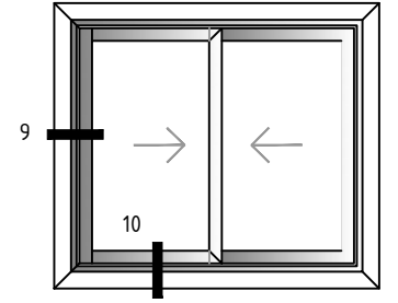
pervaz detayları jamb details
