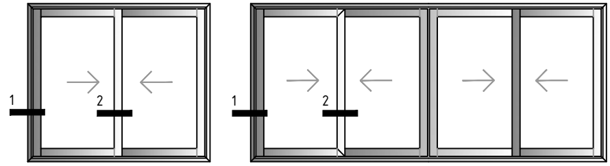
2 raylı sistem detayları Double rail system details
